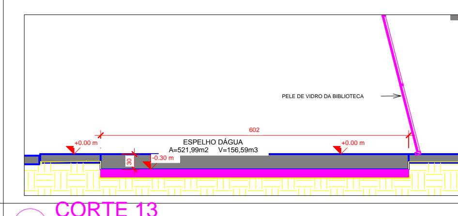
5 CORTE 13 1:50
