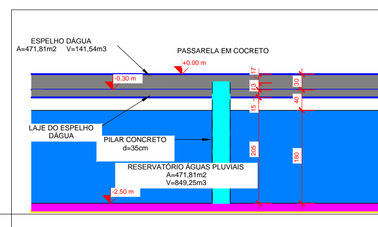
6 CORTE 14 1:50
