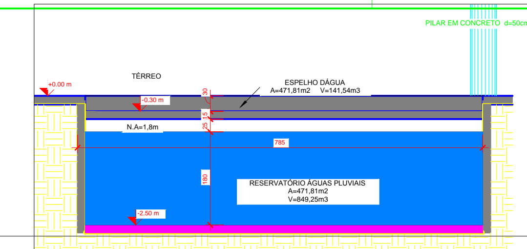
4 CORTE 12 1:50
