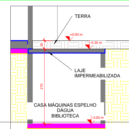
7 CORTE 15 1:50
