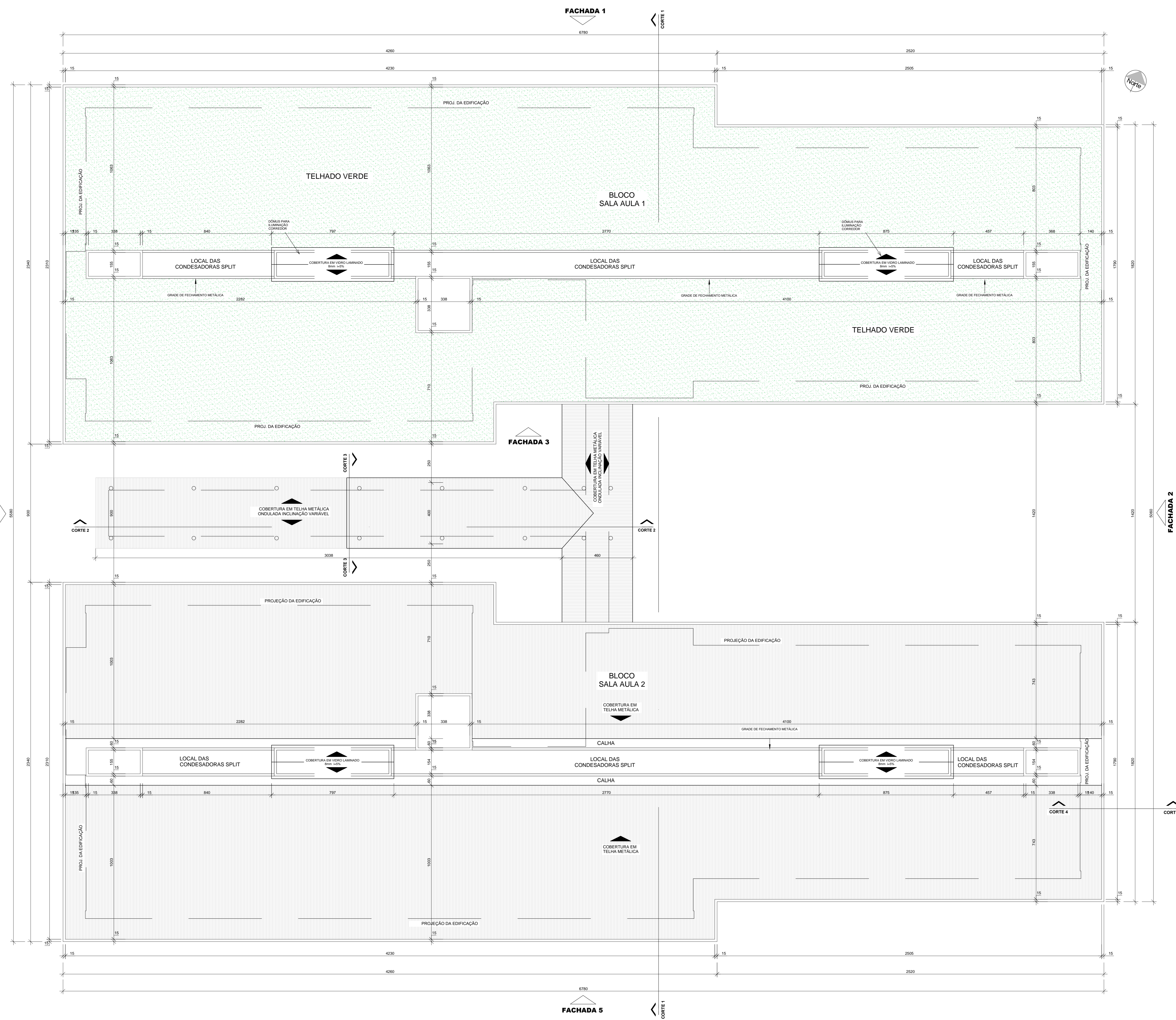
PLANTA DE COBERTURA 1 : 100
